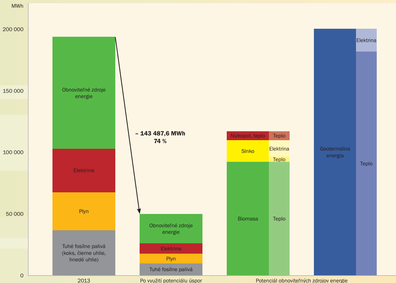
Graf 3: Porovnanie hrubej spotreby energie v Čiernohronskom MR v roku 2013 a po realizácii potenciálu úspor energie
