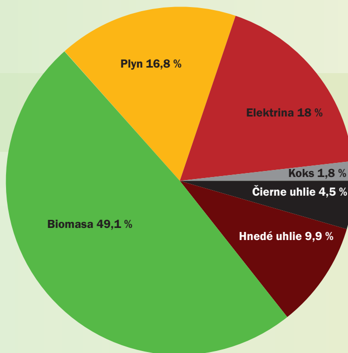
Graf 1: Podiel zdrojov energie na celkovej hrubej spotrebe energie v Čiernohronskom MR (2013)
