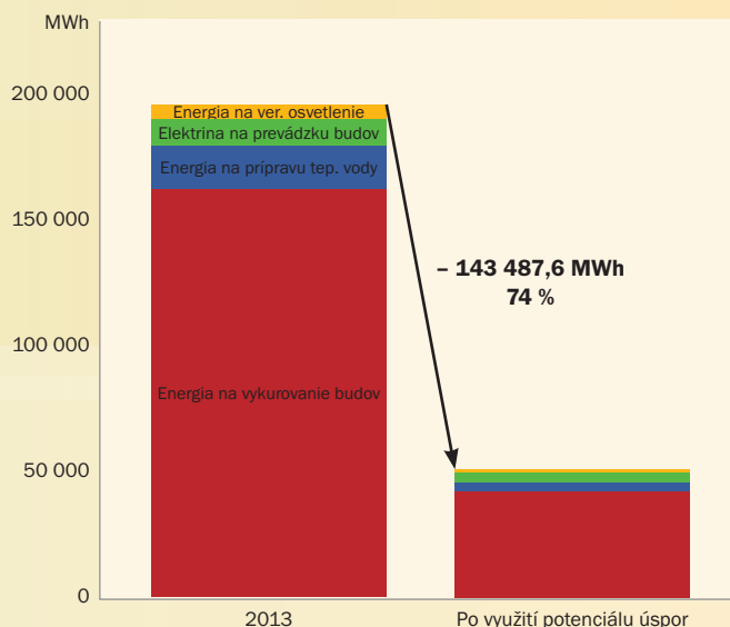
Graf 2: Porovnanie hrubej spotreby energie v Čiernohronskom MR v roku 2013 a po realizácii potenciálu úspor energie
